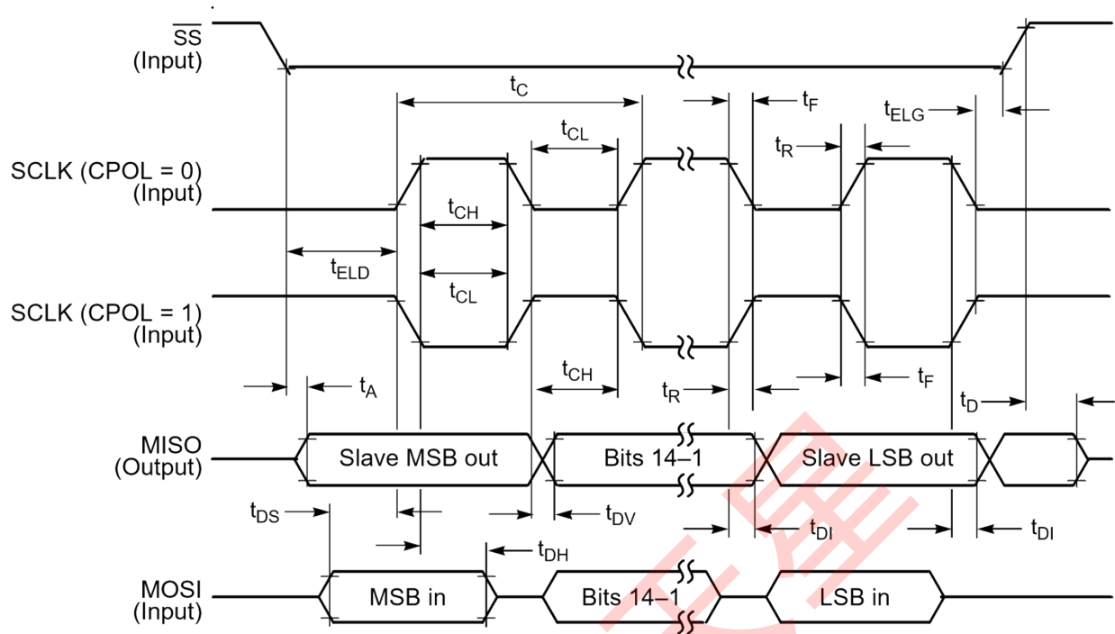
图 10-9 SPI 从属时间 (CPHA = 0)
