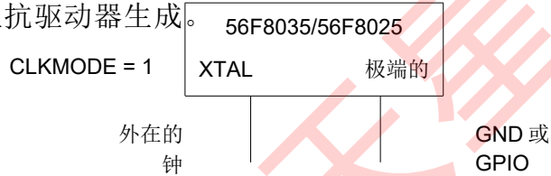
图 3-3 使用 XTAL 连接外部时钟信号
