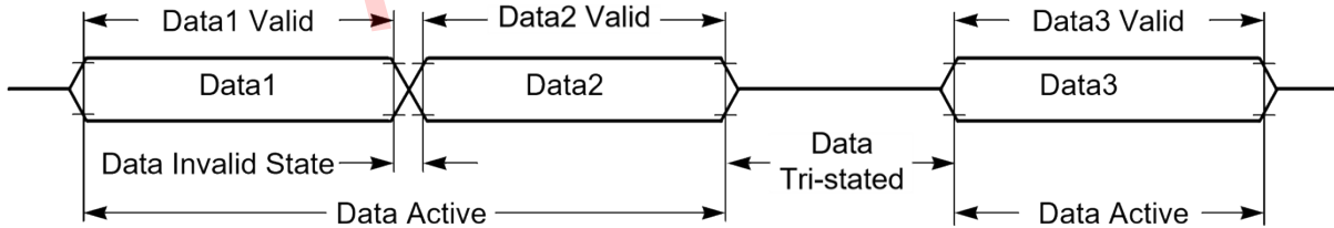
图 10-3 信号状态
