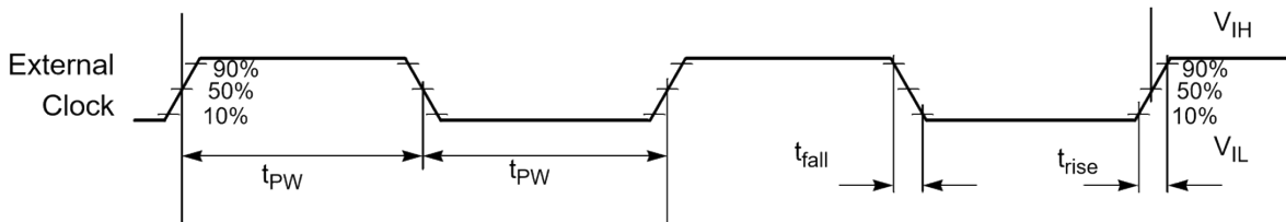
图 10-4 外部时钟定时
