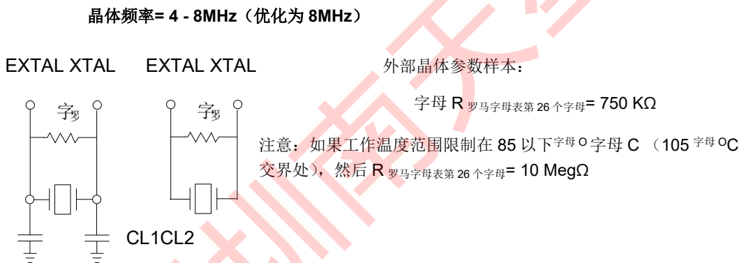
图 3-1 外部晶体振荡器电路
