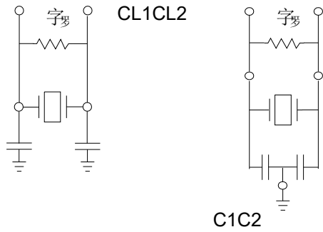
图 3-2 外部陶瓷谐振器电路
