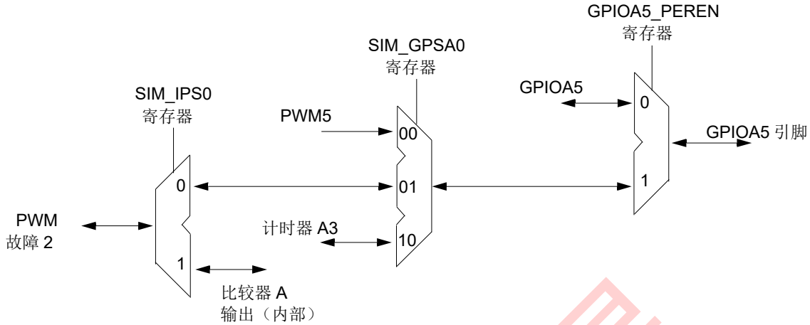
图 6-24 使用 SIM_IPS 对信号源的总体控制 第十四个英文字母控制
