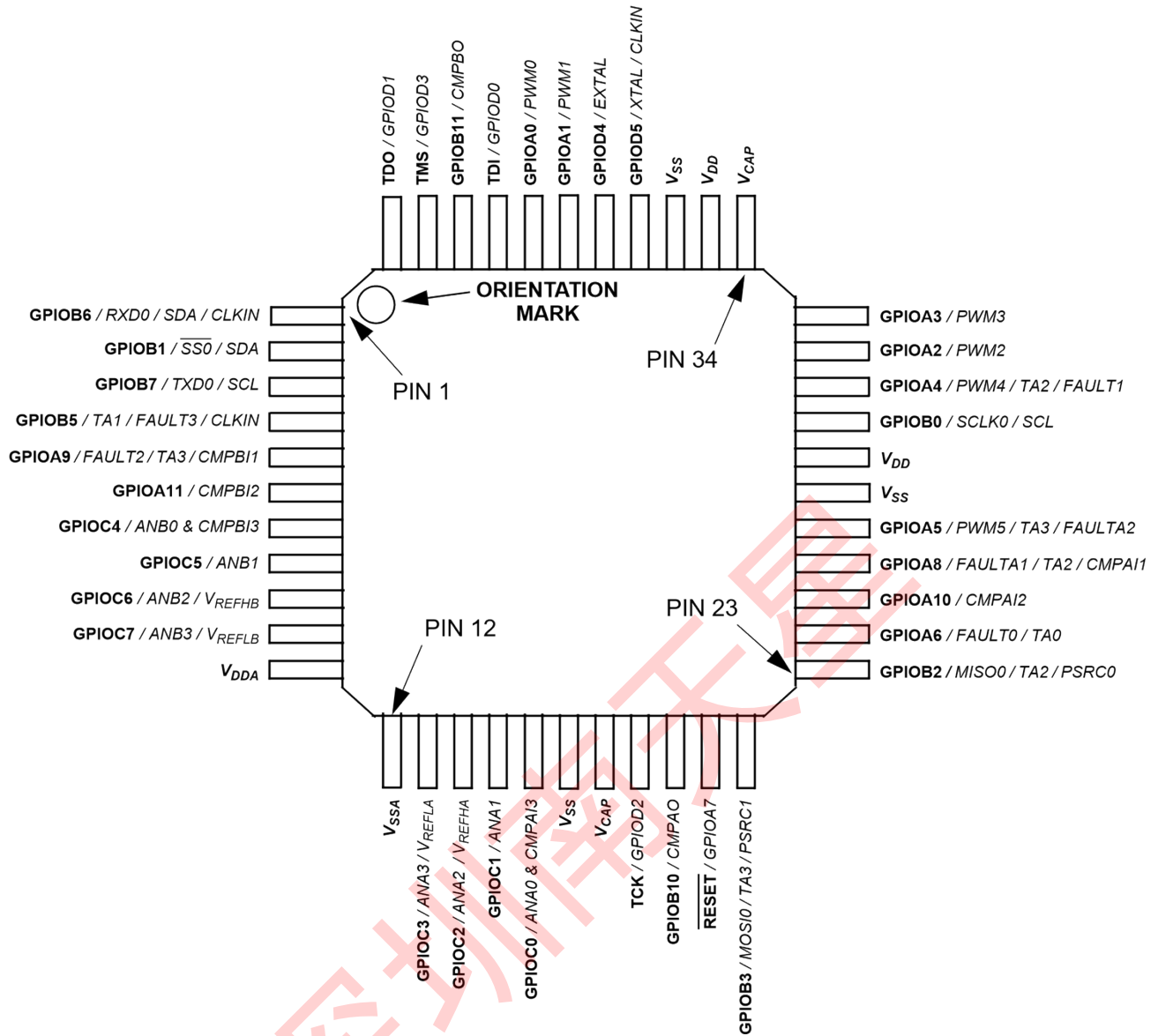
图 11-1 顶视图，56F8035/56F8025 44 针 LQFP 封装
