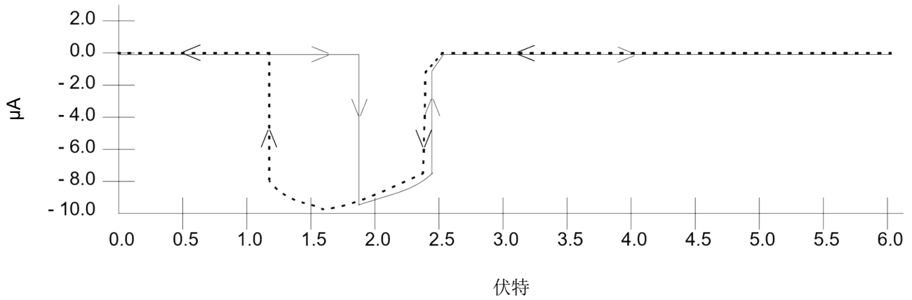
图 10-1 I DD1 盎司 Vs. V DD1 (典型; 上拉禁用)
