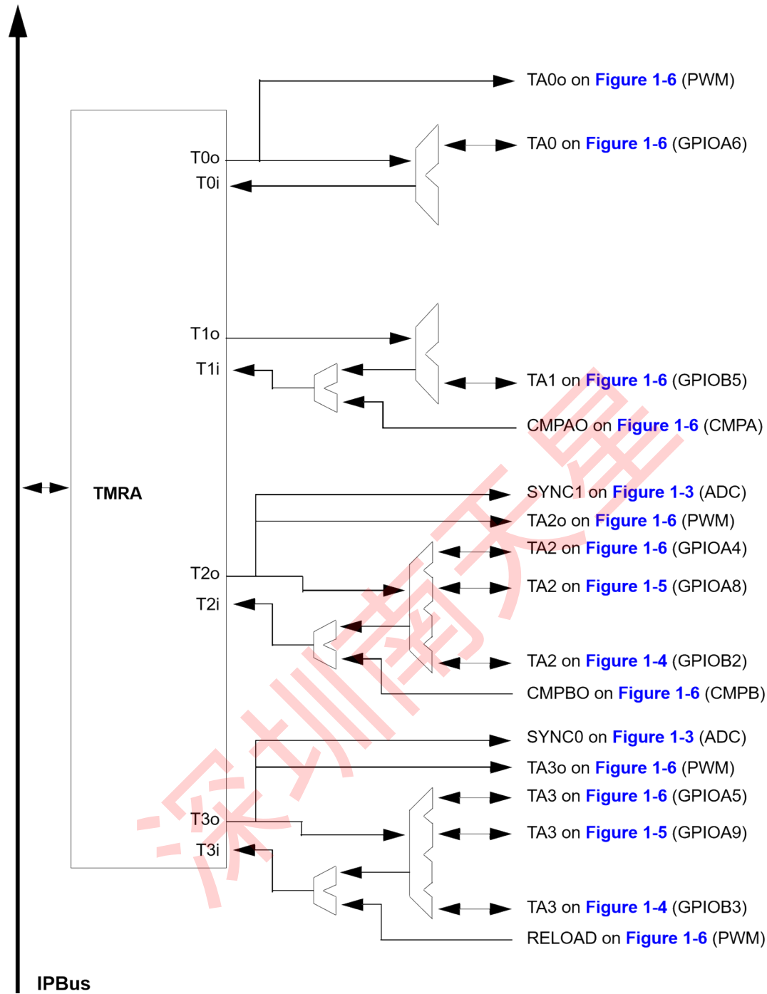
图 1-7 56F8035/56F8025 I/O 引脚输出 Muxing (第 5/5 部分)
