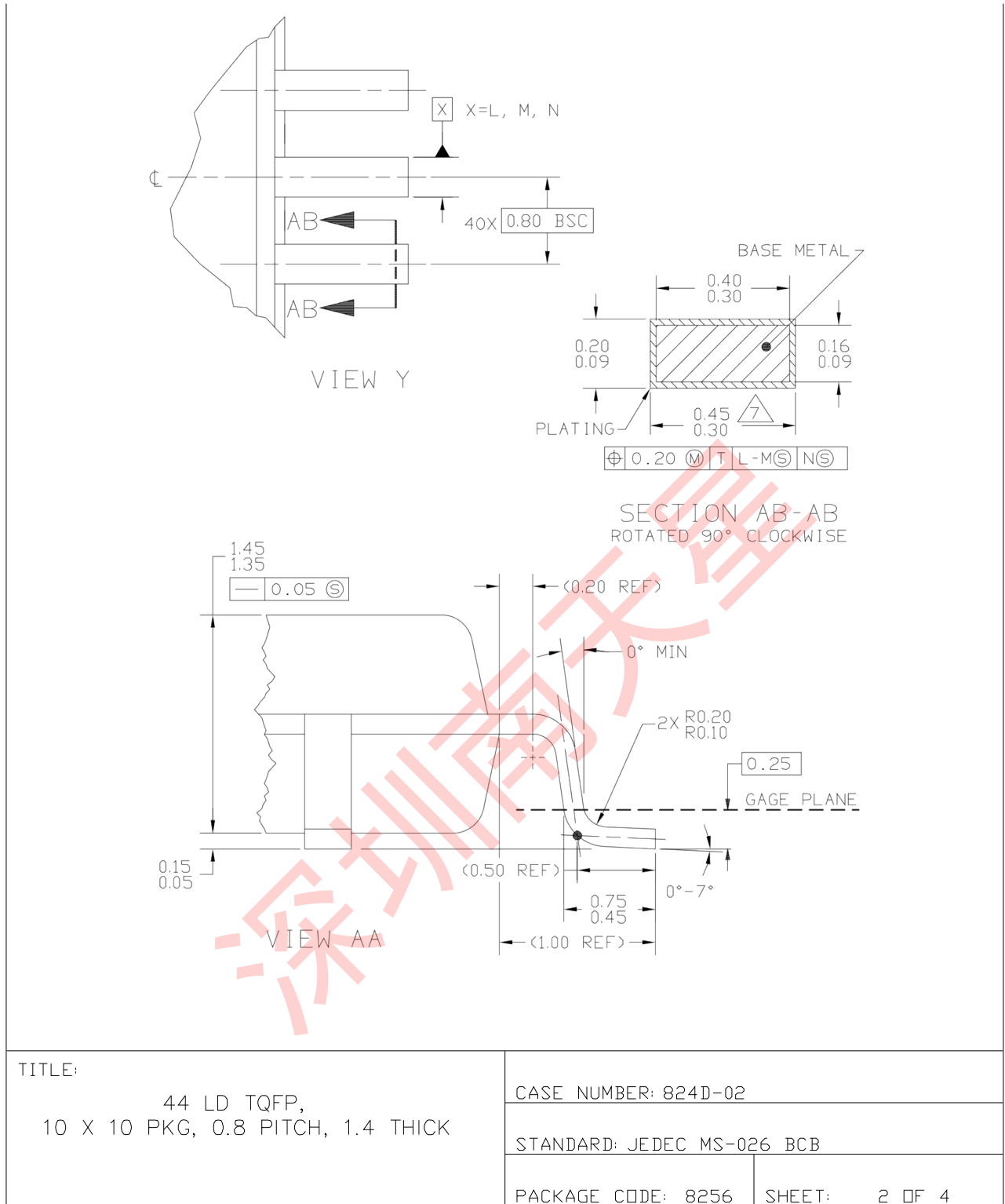
图 11-3 56F8035/56F8025 44 针 LQFP 机械信息 (2/3)
