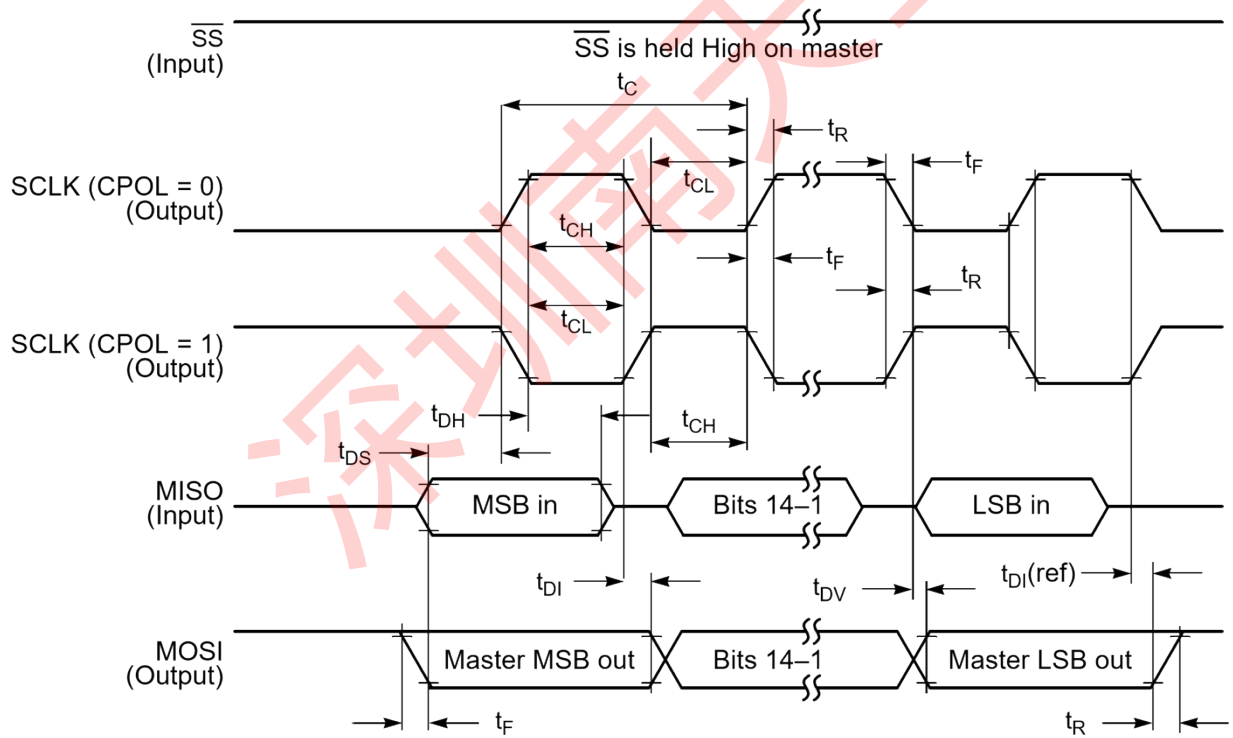
图 10-7 SPI 主计时 (CPHA = 0)
