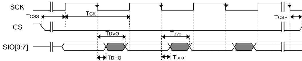
图 40. SDR 模式下的 FlexSPI 输出时序
