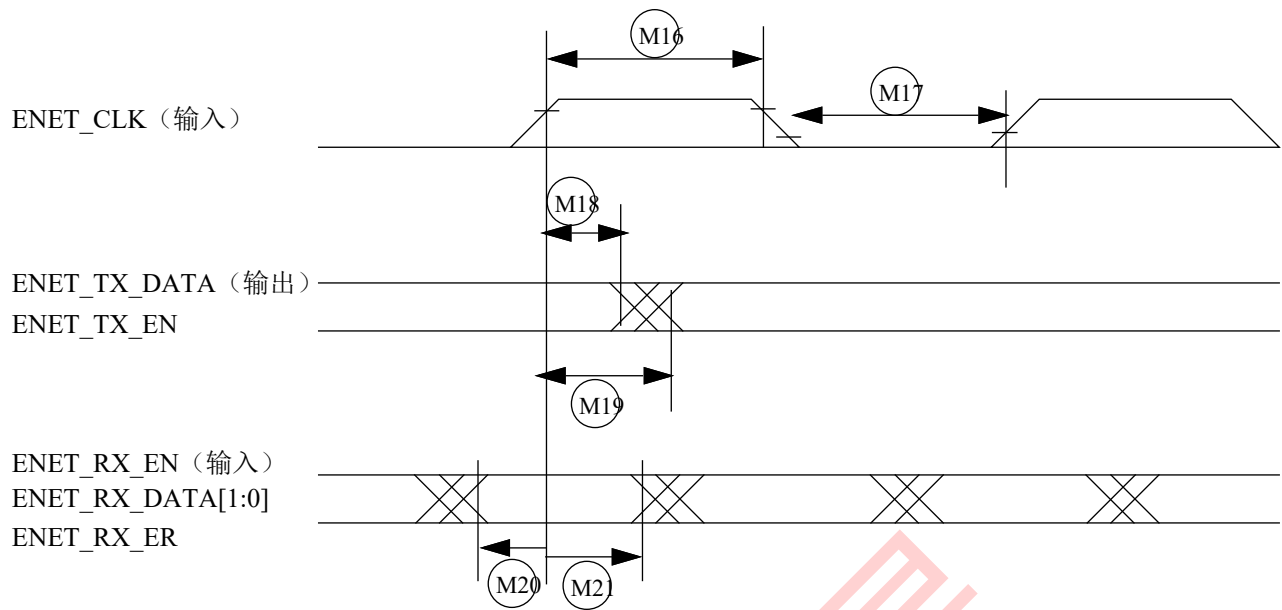
图 18. RGMII 模式信号定时图
