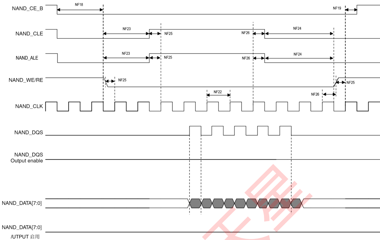
图 29。源同步模式数据读取时序图
