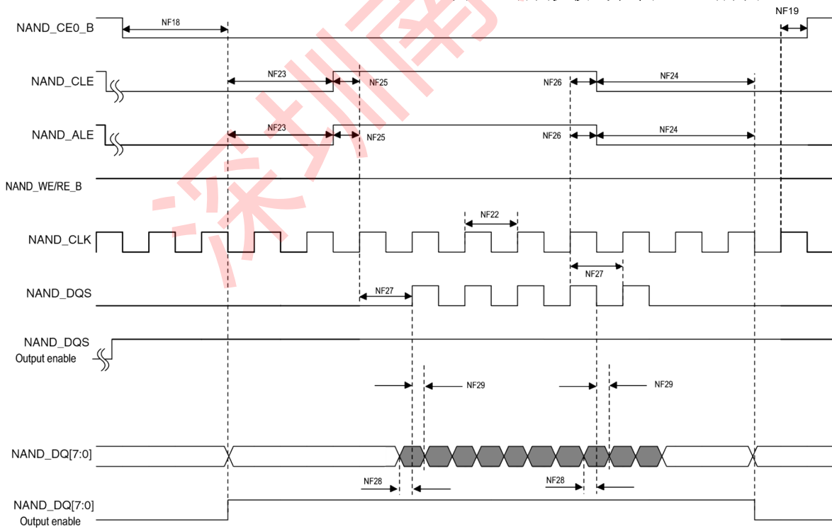
图 28。源同步模式数据写入时序图
