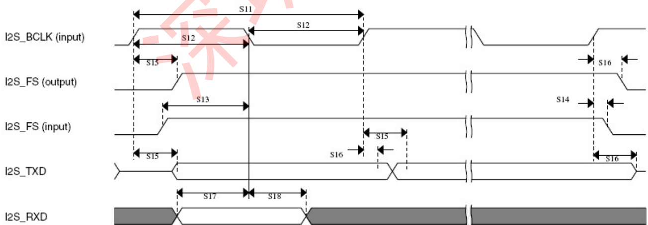
图 43. SAI 时机-从属模式
