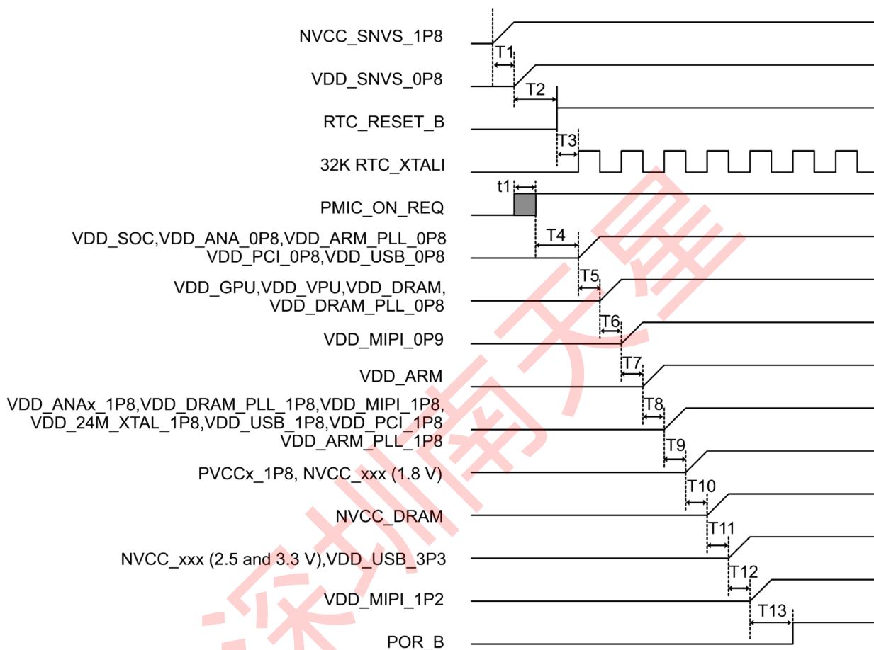
图 3. 开机序列
