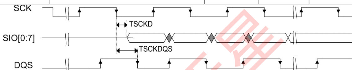
图 39. DDR 模式下的 FlexSPI 输入定时, 其中 FlexSPI 第十四个英文字母_MCR0[RXCLKSRC] = 0x3
