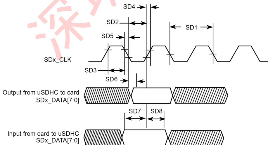
图 13. SD3.0/eMMC5.1 (SDR) 定时
