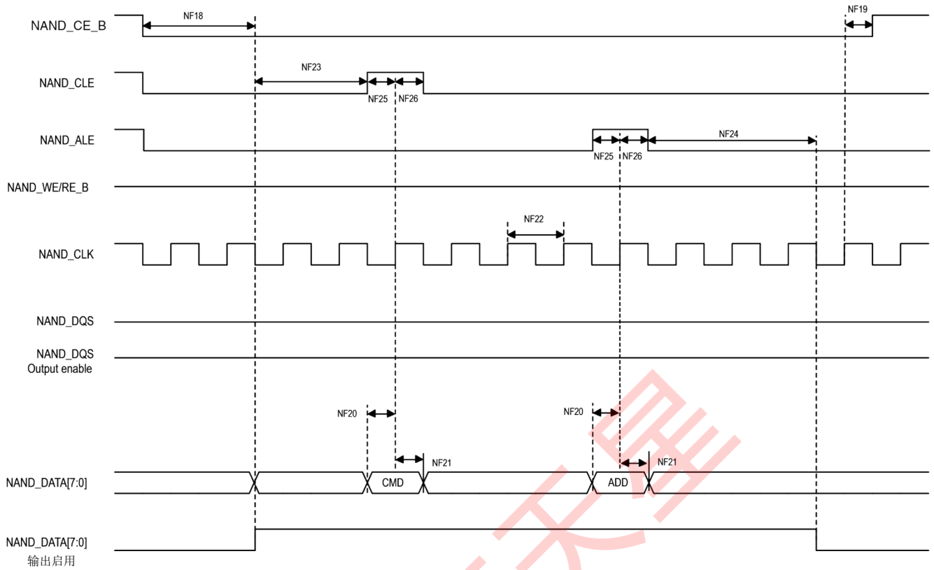
图 27。源同步模式命令和地址时序图
