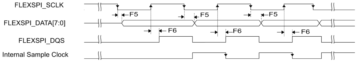
图 37. SDR 模式下的 FlexSPI 输入时序，其中 FlexSPI 第十四个英文字母_MCR0[RXCLKSRC] = 0x3（案例 A2）
