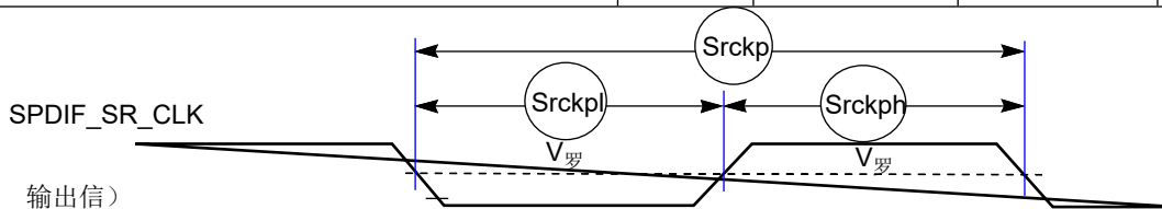
图 44. SPDIF_SR_CLK 定时图
