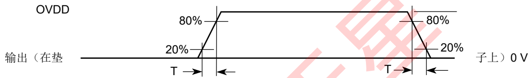
图 7. 输出转换时间波形
