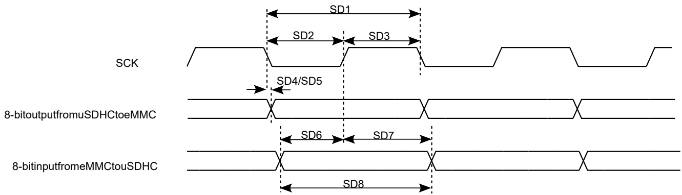
图 17. SDR50/SDR104 定时
