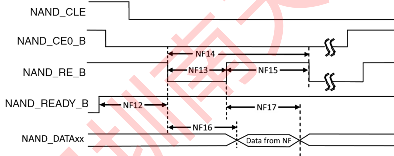
图 26. 读取数据门锁周期时序图 (EDO 模式) 表 40. 异步模式定时参数 1
