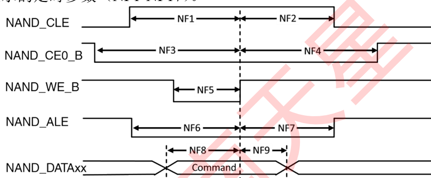
图 22。命令门锁周期正时序图
