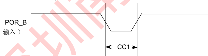
图 9. 重置时序图
