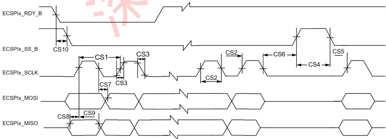
图 11. ECSPI 主模式定时图
