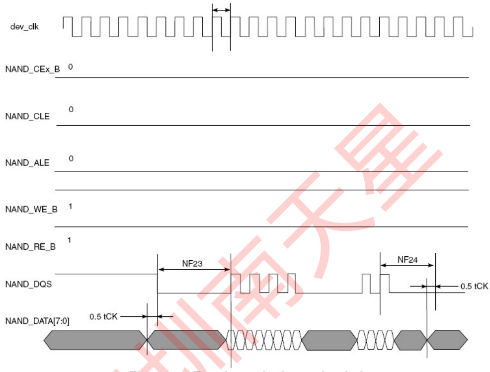
图 31。切换模式数据写入时序
