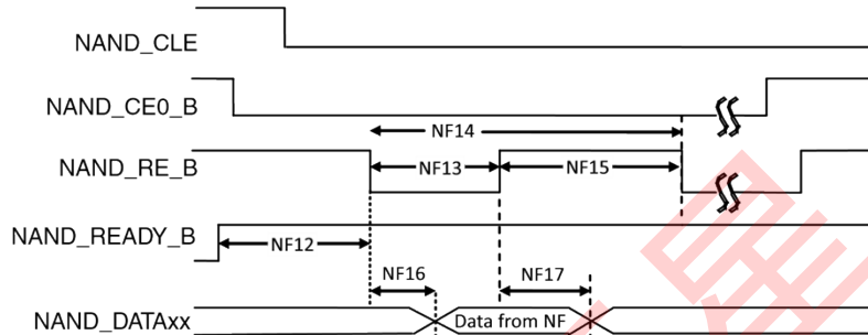
图 25. 读取数据门锁周期定时图 (非 EDO 模式)
