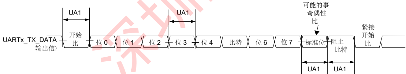
图 46. UART RS-232 串行模式传输时序图
