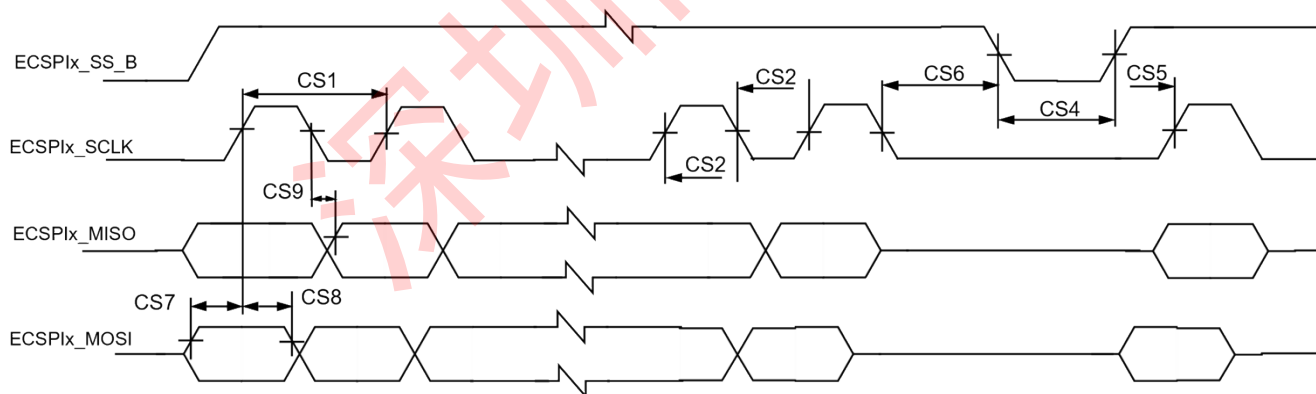
图 12. ECSPi 从模式定时图
