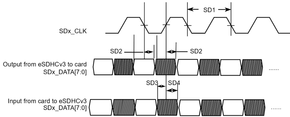
图 14. eMMC5.1/SD3.0 (DDR) 计时
