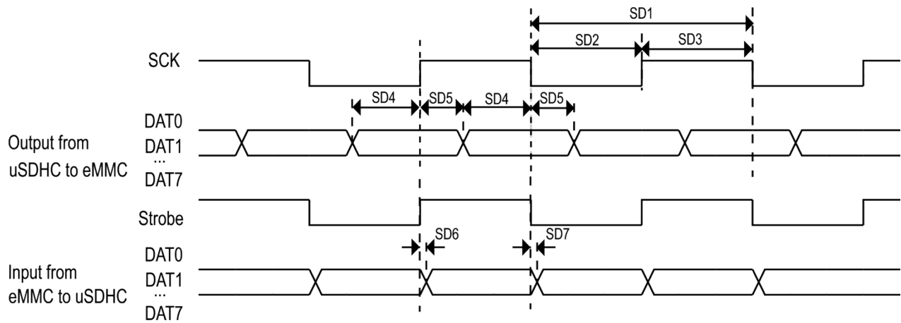
图 15. HS400 计时
