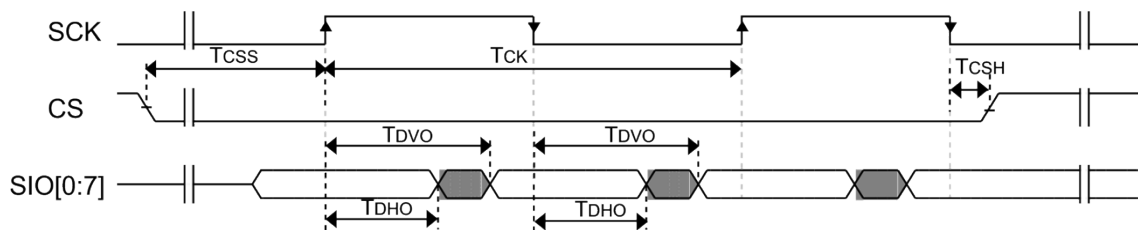
图 41. DDR 模式下的 FlexSPI 输出计时
