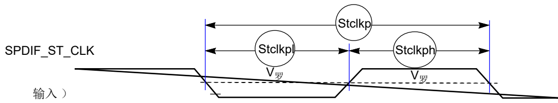
图 45. SPDIF_ST_CLK 定时图
