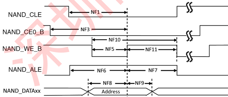
图 23。地址门锁周期定时图
