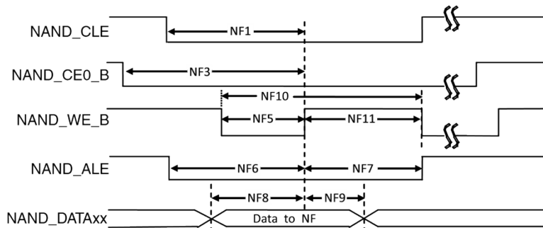
图 24. 写入数据门锁周期时序图
