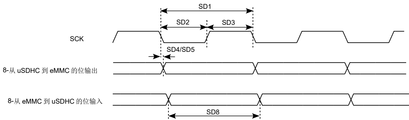
图 16. HS200 计时
