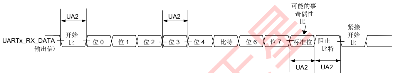
图 47. UART RS-232 串行模式接收定时图
